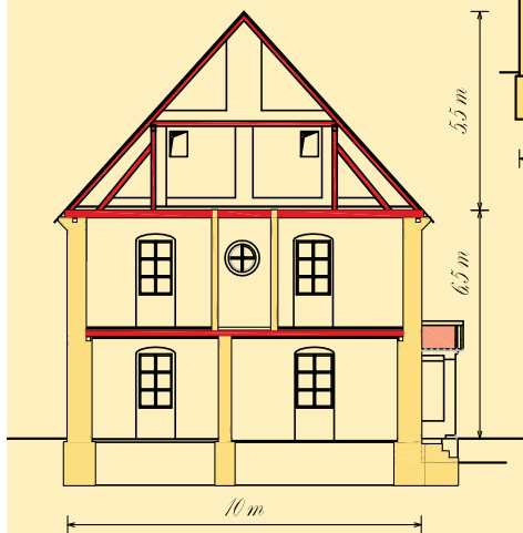
Presjek C - C
