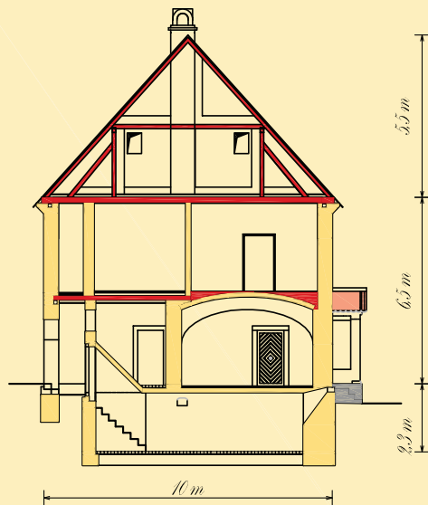
Presjek A - A
