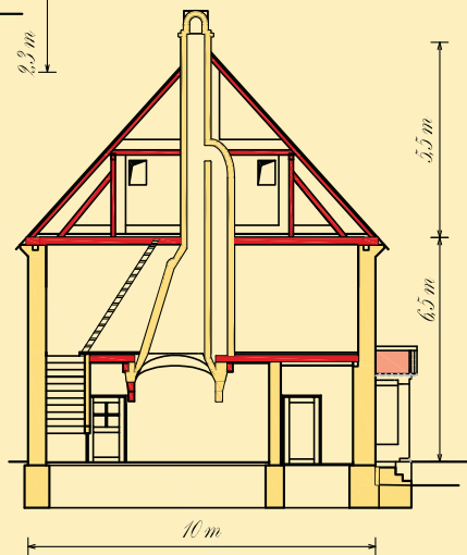
Presjek B - B
