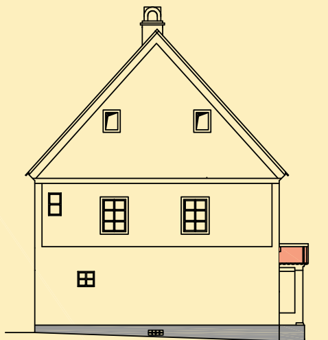
Kapadno pročelje
